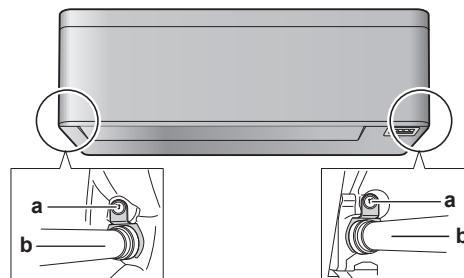
a Vijak za pričvršćivanje izolacije b Crijevo za odvod kondenzata
