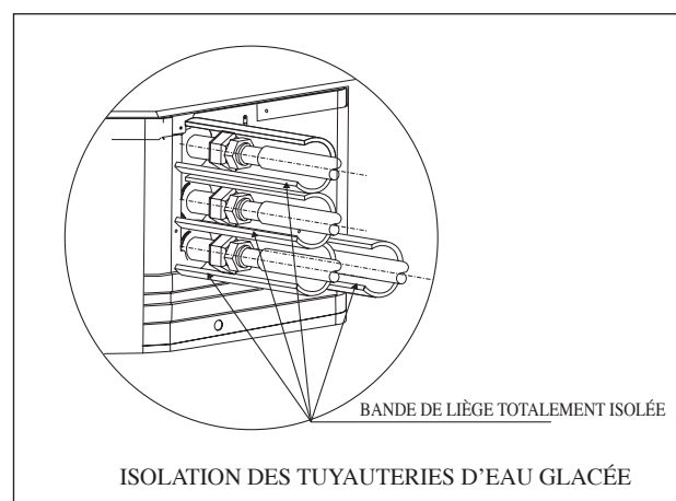
4 Système de tuyaux
