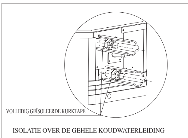
2-leidingensysteem
