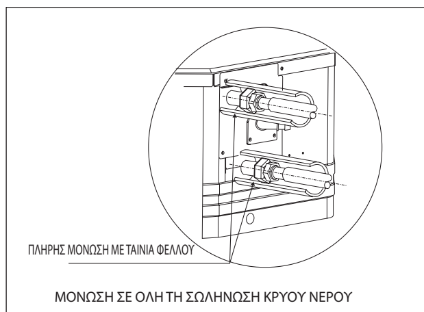
Σύστημα 2 σωλήνων
