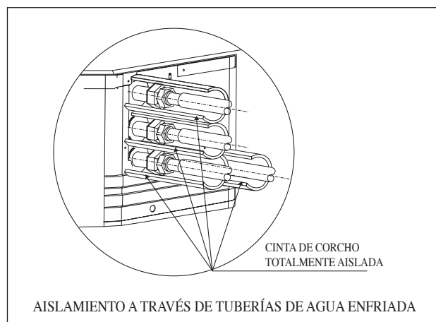
4 Tuberías sistema
