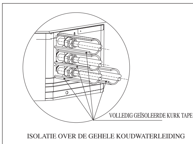
4-leidingensysteem
