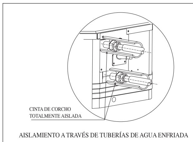
2 Tuberías sistema
