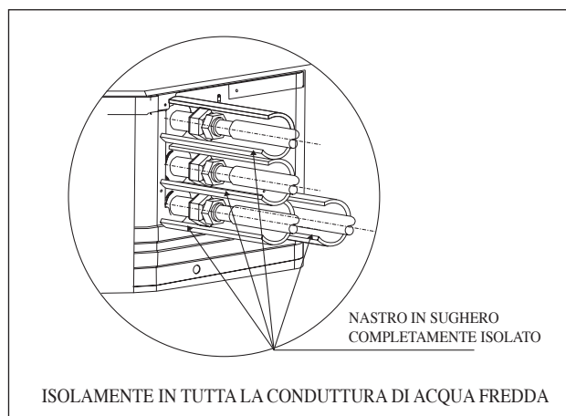
4 Tubi di sistema
