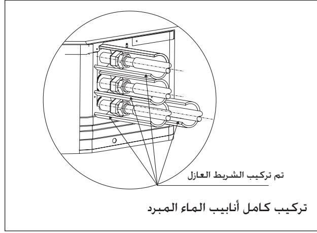
أنابيب نظام 4
