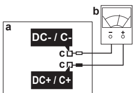
a Glavna printana ploča b Multimetar c Mjerne tačke preostalog napona
