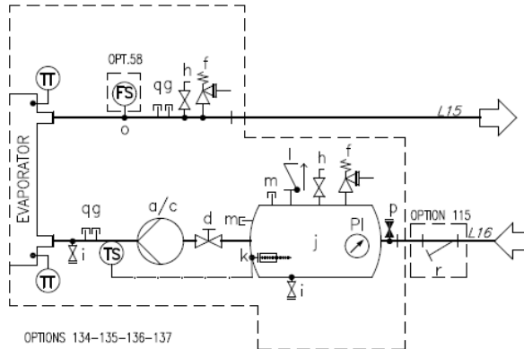
Sl. 18 – Hidraulički dijagram za jednu pumpu / dvostruku pumpu (opcija 78-79-80-81/134-135-136-137) (maks. radni tlak 6 bara)
