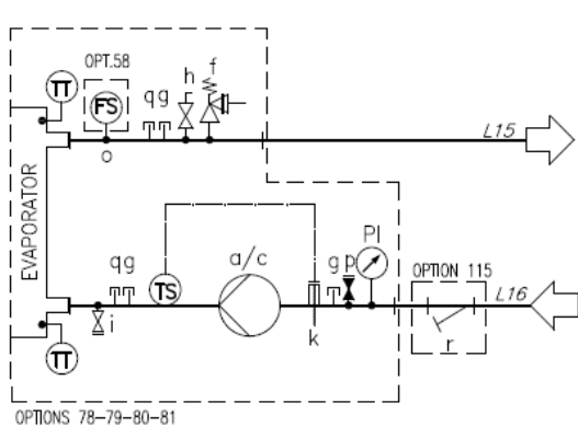
Sl. 18 – Hidraulički dijagram za jednu pumpu / dvostruku pumpu (opcija 78-79-80-81/134-135-136-137) (maks. radni tlak 6 bara)
