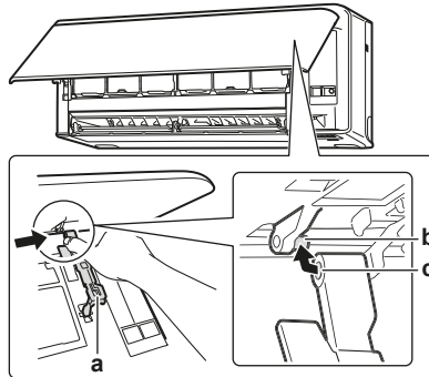
a Ručica b Osovina c Utor osovine
